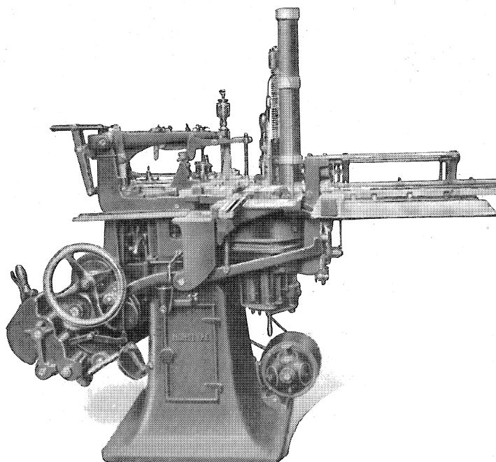
FIG. 41. — LA FONDEUSE " UNIVERSELLE ".
