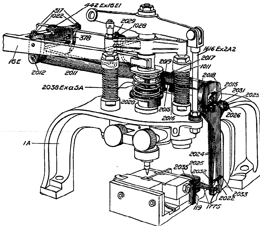
FIG. 39. — APPAREIL A ESPACES BASSES.
