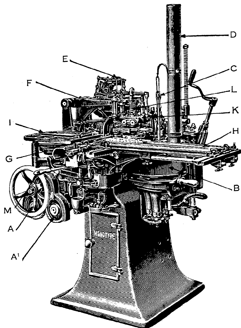
FIG. 18 — LA FONDEUSE " MONOTYPE ", VUE DE FACE.
