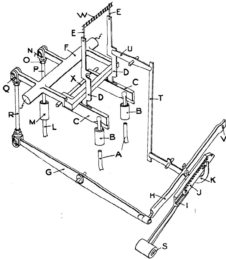
FIG. 12 — VUE PERSPECTIVE MONTRANT LES ORGANES DE COMMANDE DES POINÇONS ET DE CONTRÔLE DE LA CRÉMAILLÈRE DES UNITÉS.
