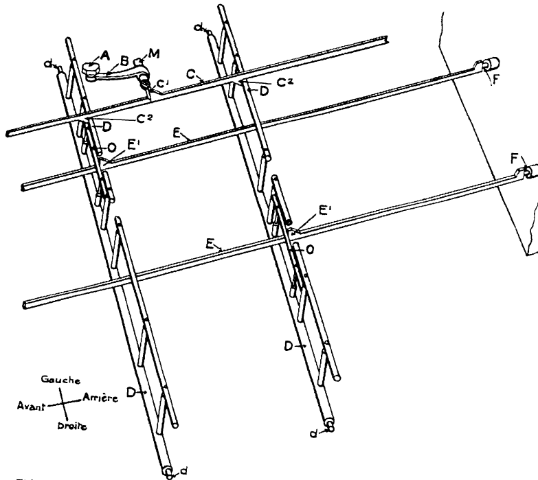
FIG. 10. — VUE PERSPECTIVE MONTRANT L'ACTION D'UNE TOUCHE SUR LA LAME INTERMÉDIAIRE CORRESPONDANTE, QUI SÉLECTIONNE LES VALVES VOULUES.
