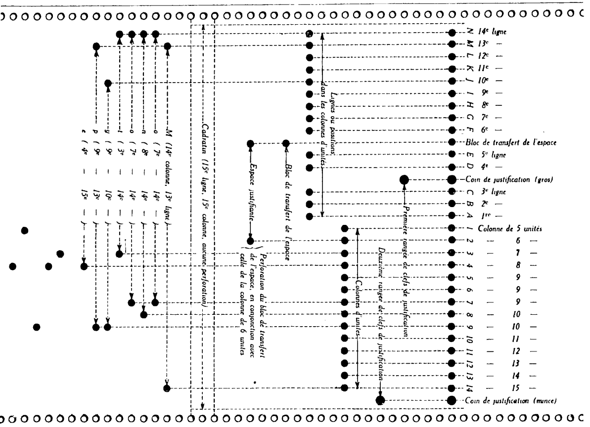
FIG. 9. — RÉPARTITION ET DÉSIGNATION DES PERFORATIONS SUR LA BANDE DE PAPIER
