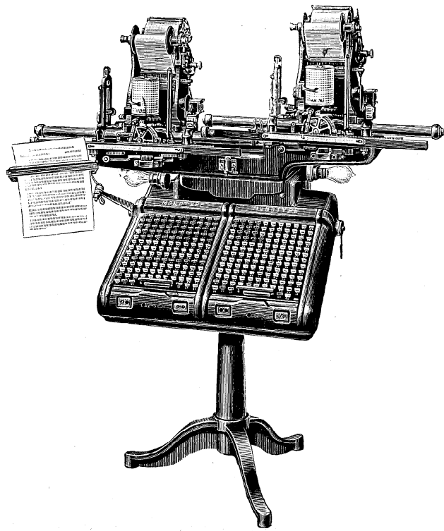
FIG 2 — LE CLAVIER " MONOTYPE " MODÈLE " DD "
