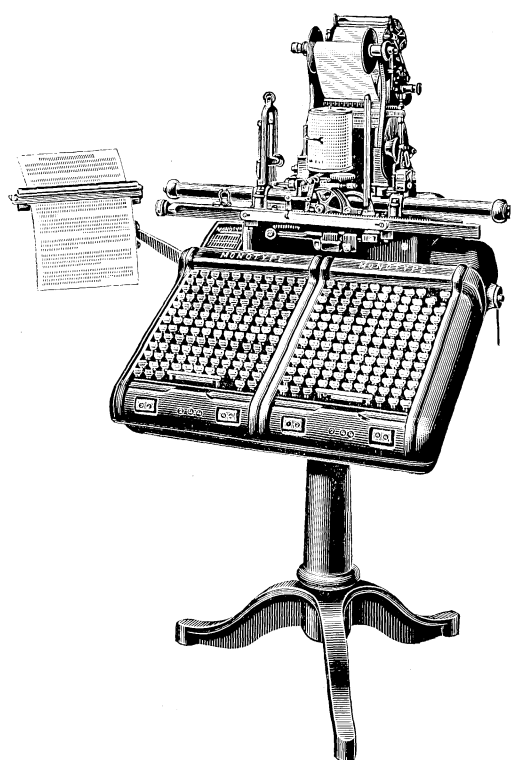
FIG. 1. — LE CLAVIER " MONOTYPE " MODÈLE " D ".
