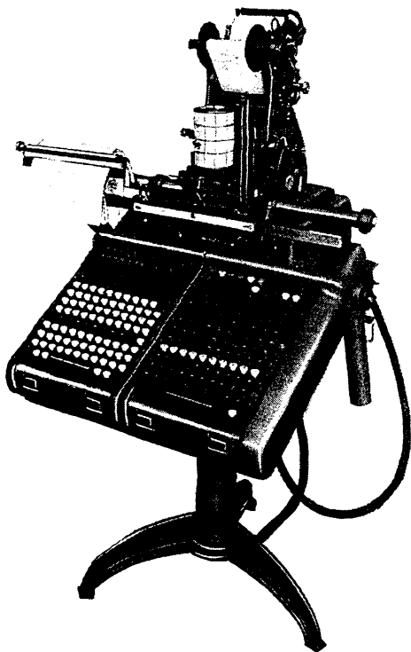
» Monotype « Normal-Setzmaschine
